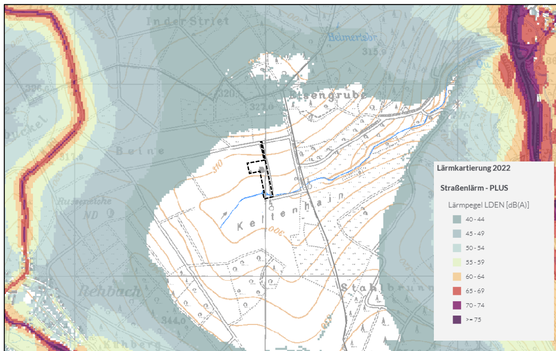
Abbildung 9: Lärmpegel LDEN (tags)
